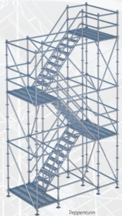
Treppenturm
